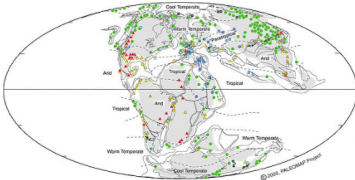
Das Weltklima in Unterer Kreide (nach Scotese)
